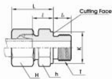
Form B stud end
