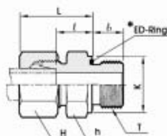
Form E stud end
