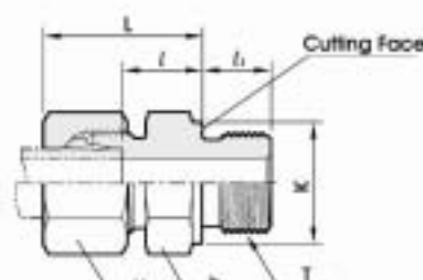
Form B stud end
